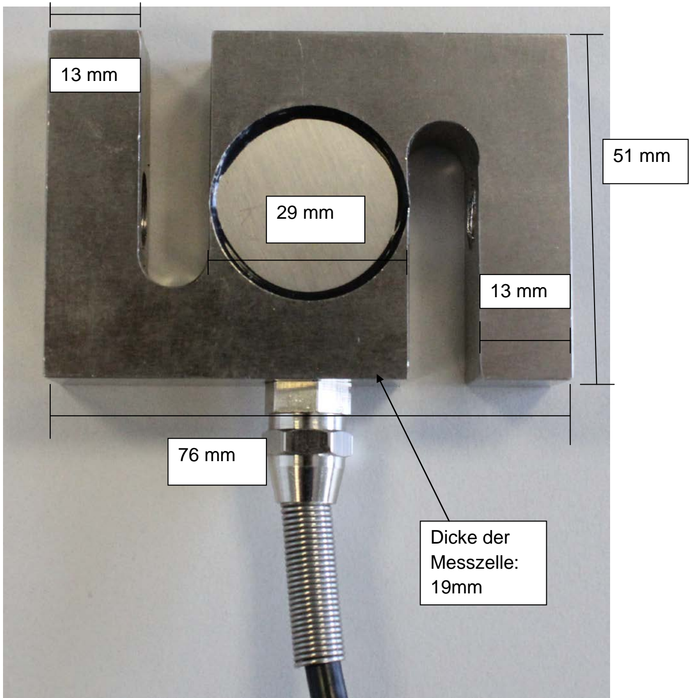
Externe Messzelle FL 2K
